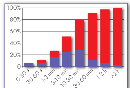
Rys. 8. Czas połączenia z ASG-EUPOS podczas pojedynczego logowania (na czerwono – statystyka skumulowana)
